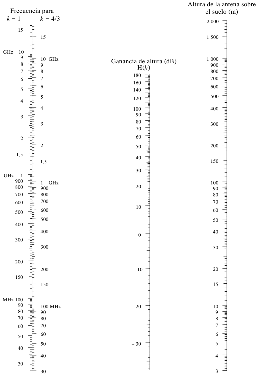
FIGURA 4-b Difracción para una tierra esférica – Ganancia de altura
